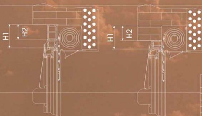
montaža na prozor sa dodatnim profilom
